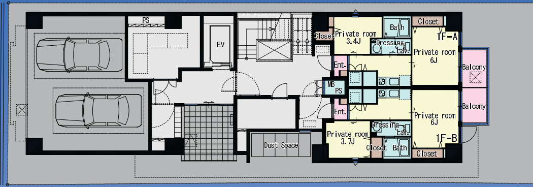
1F Plan 1:100
